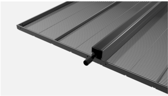
——简洁轻盈—— 哑黑色箱体设计、电源梁仅宽52mm，内置卡扣连接件、外观无螺丝搭扣，干净整洁。
